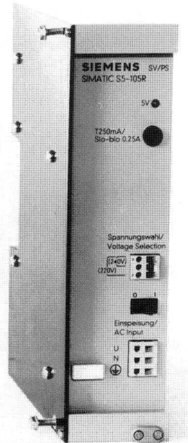
Bild 9 Stromversorgungsbaugruppe 220/240 V AC
