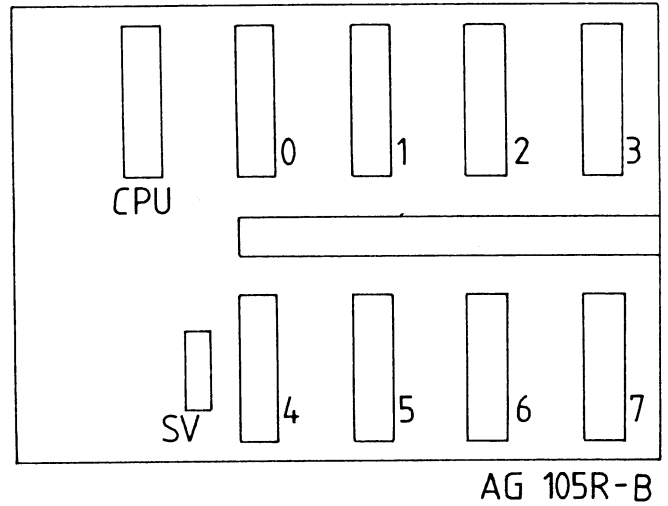
Bild 18 Anordnung der Stecker auf der Rückwandplatine
