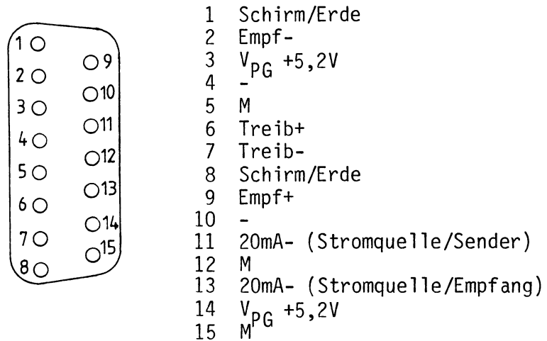
Bild 19 Schnittstellenbelegung zum PG 605R
