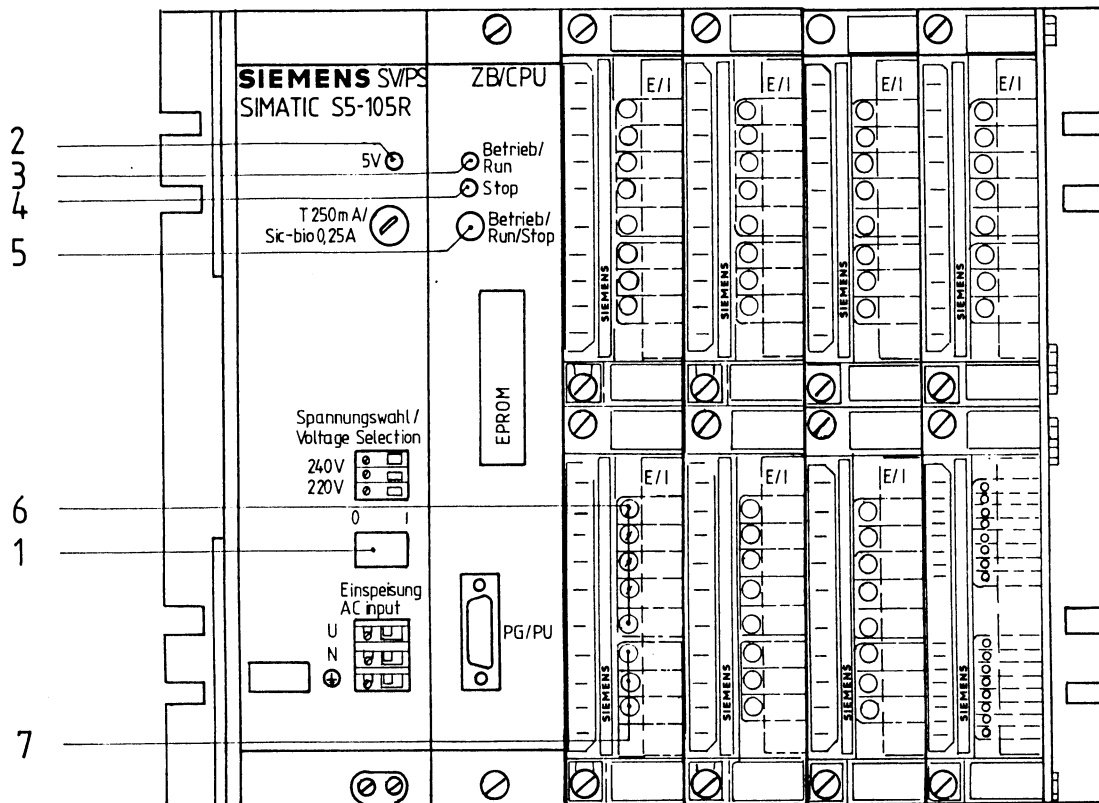
Bild 16 Bedien- und Anzeigeelemente des AG 105R-B
