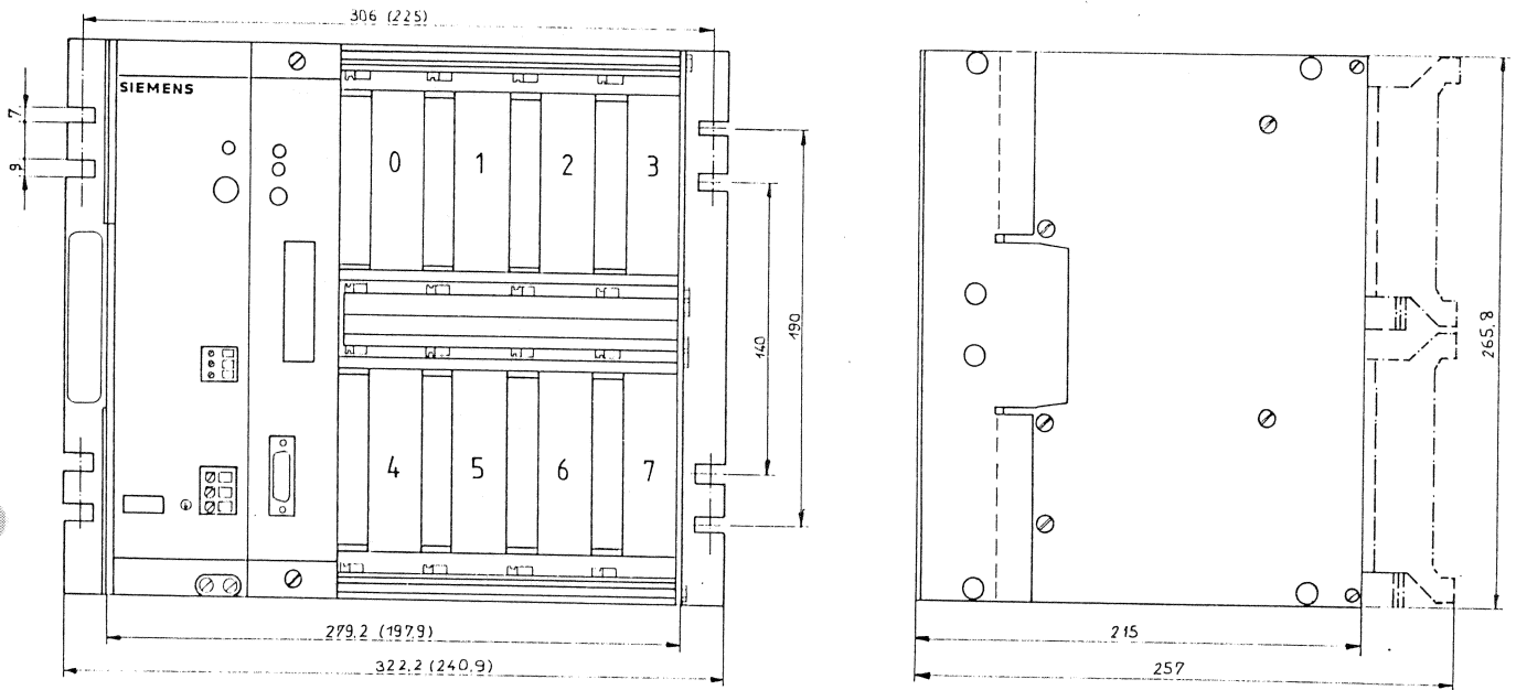
Bild 7 Maßbild des AG 105R-B (Maße in Klammern gelten für AG 105R-A)
