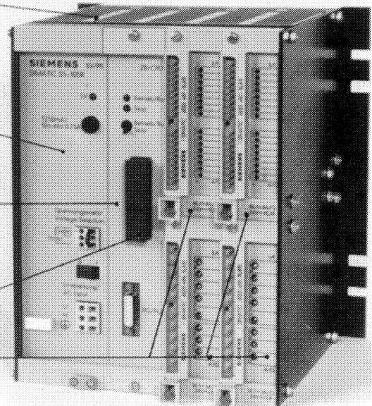
Bild 3 Automatisierungsgerät 105R-A vollständig bestückt
