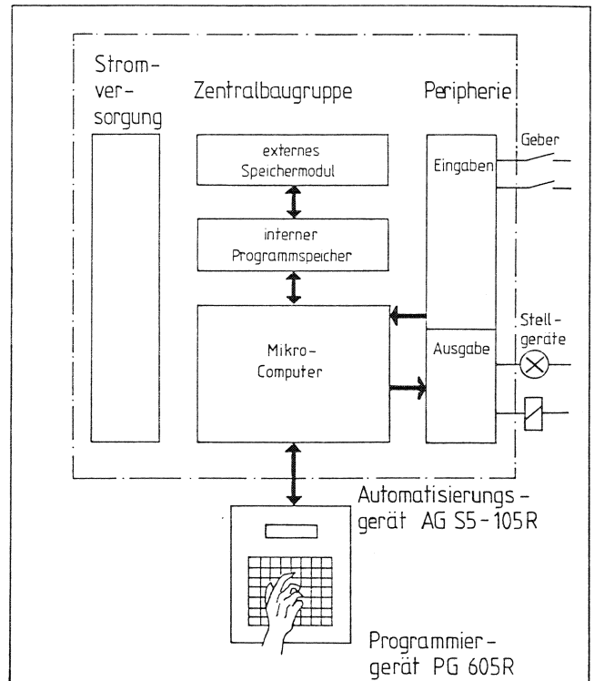
Bild 4 Blockschaltbild des AG 105R
