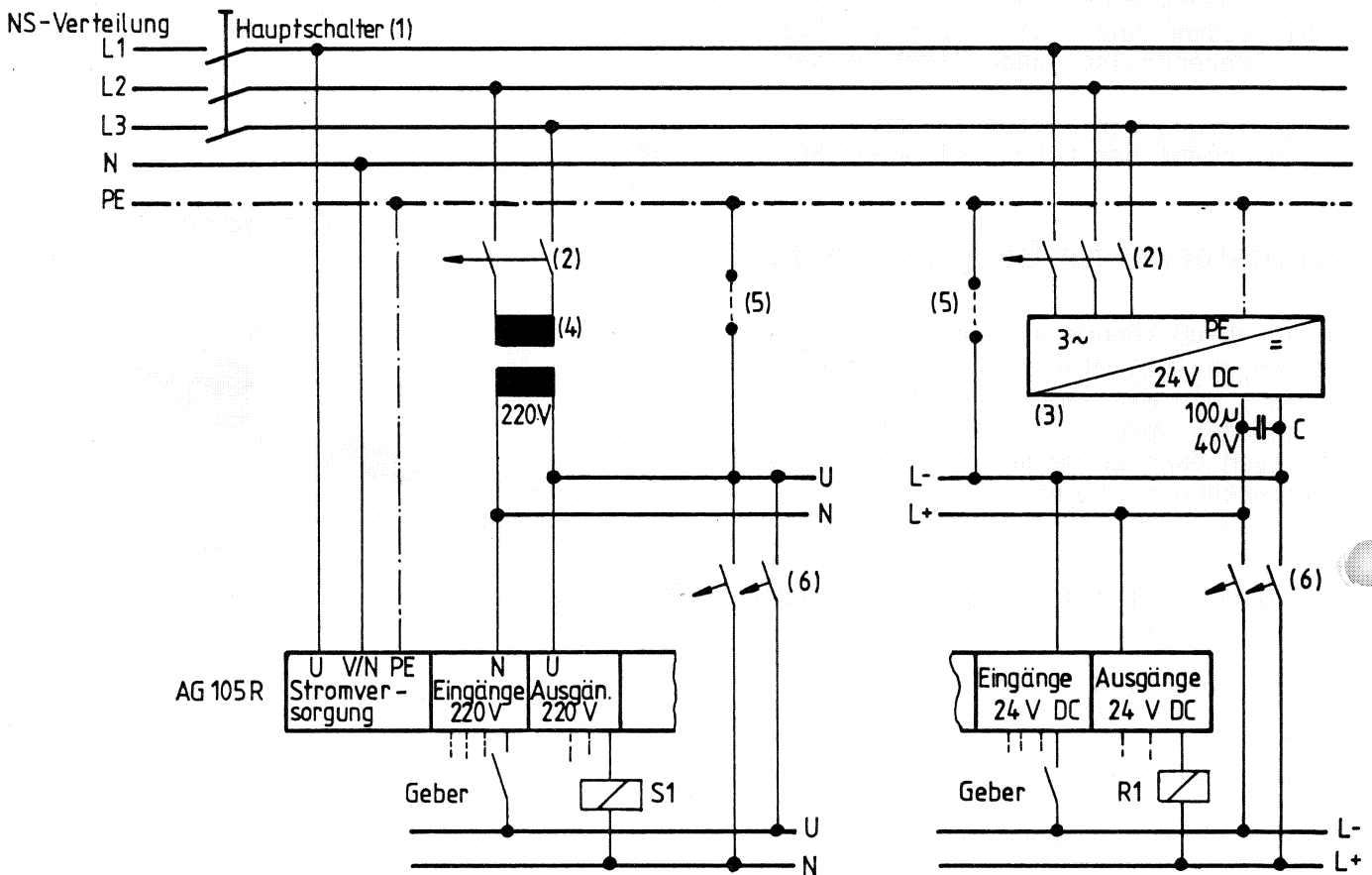
Bild 15 Aufbauvorschlag des AG 105R
