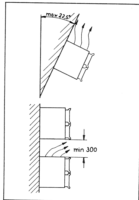
Bild 8 Montagemöglichkeiten
