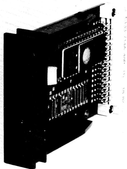
Bild 23 EPROM-Speichermodul
