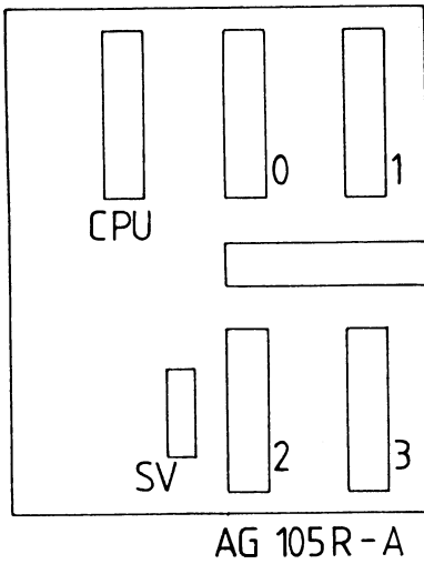
Bild 18 Anordnung der Stecker auf der Rückwandplatine
