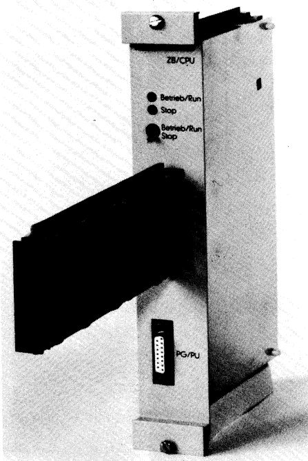
Bild 22 Zentralbaugruppe mit gestecktem Programmieradapter und Speichermodul
