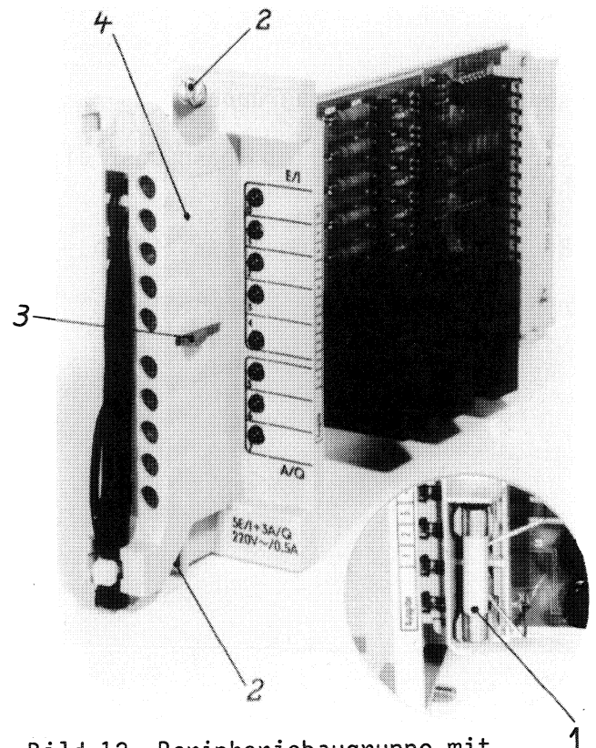
Bild 12 Peripheriebaugruppe mit Frontstecker
