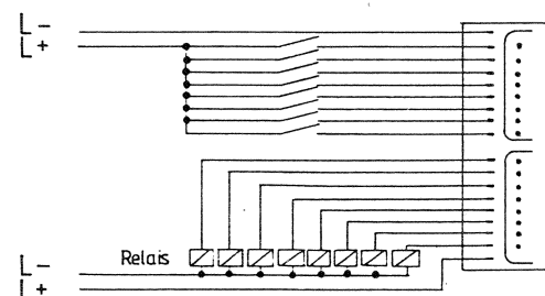
Bild 14 Verdrahtung der Peripheriebaugruppen
