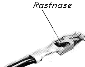
Bild 13 Mini-Spring-Kontakt
