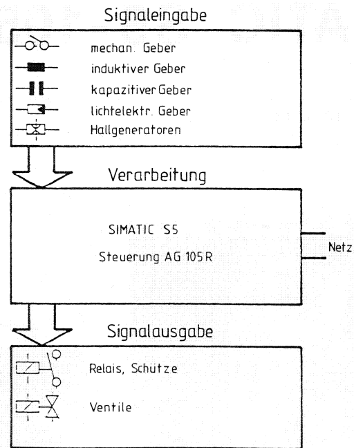
Bild 2 Einsatz des Automatisierungsgerätes 105R
