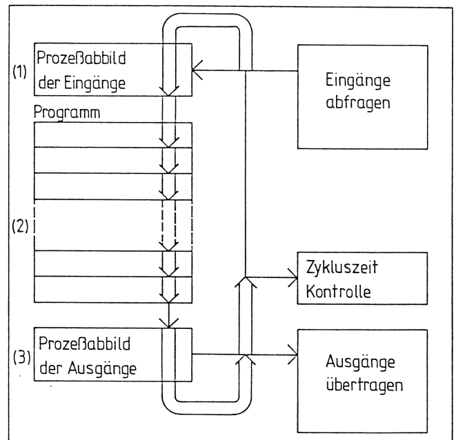
Bild 6 Arbeitsweise des AG 105R
